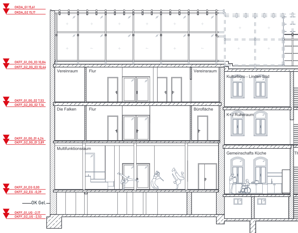
Schnitt A-A
