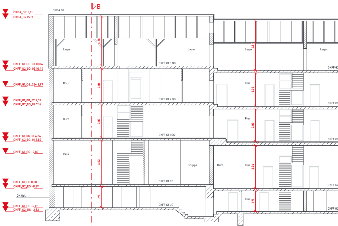
Schnitt A-A
