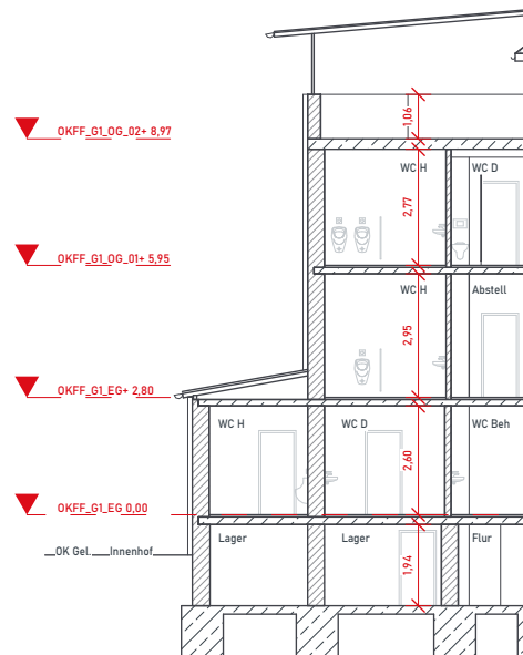
Schnitt B-B
